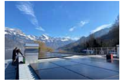
Das neue Solardach der sagibeiz
